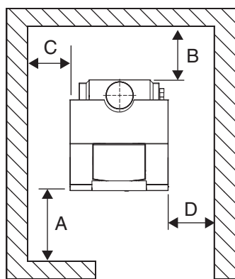
Рис. 7 Рекомендуемые расстояния от стен [мм] (в скобках указаны минимальные размеры)
