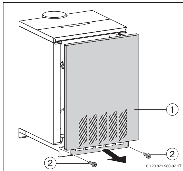
Рис. 37 Установка передней стенки котла
